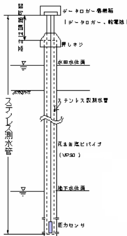
水田用水位計設置例
